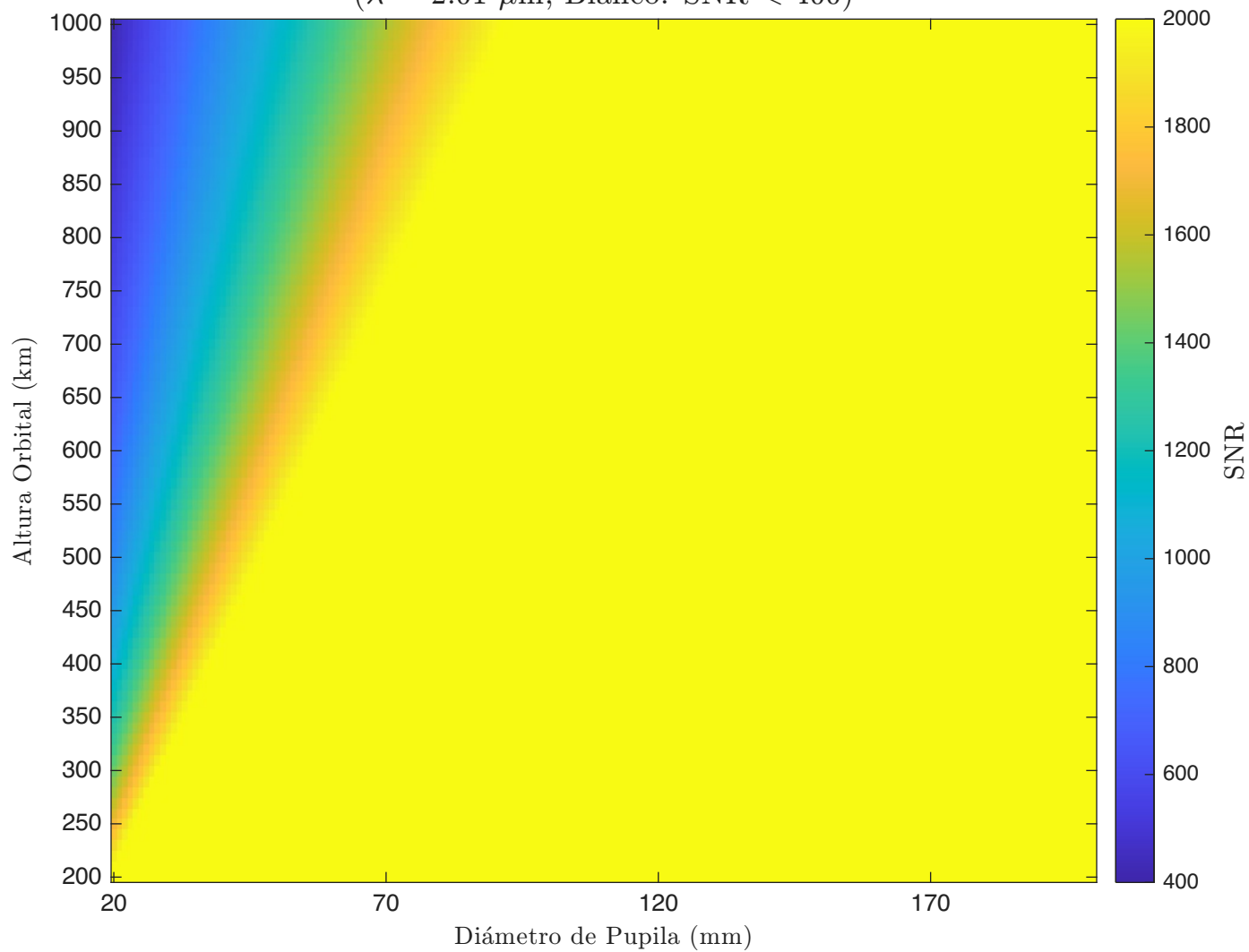
SNR - Refractivo - Detector 2 ( \lambda = 2.01 \mu\text{m} , Blanco: SNR < 400)
